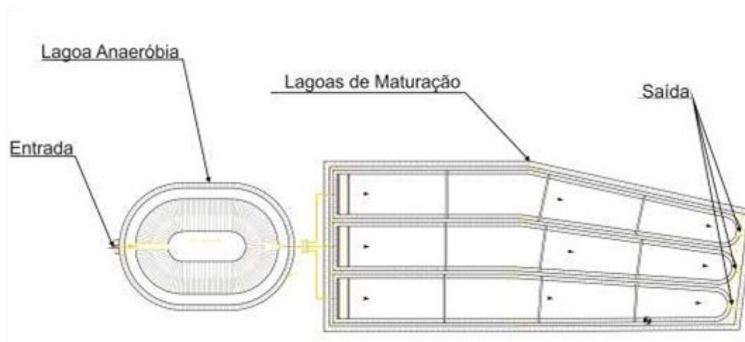
Figura 24: Croqui da Estação de Tratamento de Efluente Catuípe.
